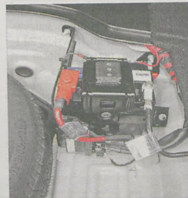
Urządzenie doładowujące akumulator przy dłuższych postojach np. w korkach – dzięki niemu będzie cały czas działać klimatyzacja czy grać radio.
