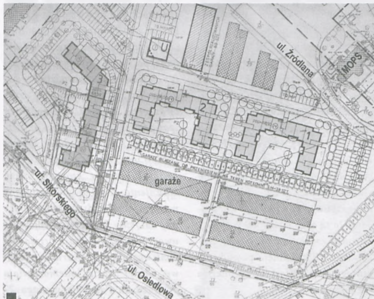
Kolorem ciemnoszarym zaznaczyliśmy blok znajdujący się obecnie w budowie (3). Kolorem jasnoszarym wskazujemy planowane bloki (1 i 2).
