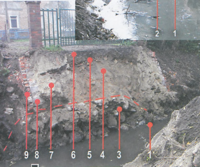
Strumień Junikowski – brzeg wschodni, z tyłu Dom Włodarza; 1 – pal wschodni, 3 – grobla kamienna z ok. 1330 r. (zaznaczona przerywaną linią), 4 – grobla ziemna z ok. 1444 r., 5 – warstwa tłuczonej cegły z ok. 1870 r., 6 – nawierzchnia gruntowa, 7 – wypełnienie piaskowe z 1992 r., 8 – mur z bloczków betonowych z 1992 r., 9 – obmurowanie ceglane z 1992 r.
