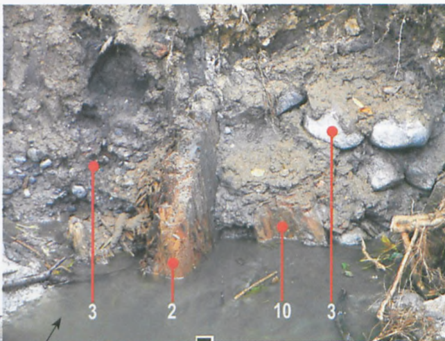
Szczegół zdjęcia brzegu zachodniego; 2 – pal zachodni, 3 – grobla kamienna z ok. 1330 r., 10 – pal boczny wspierający zastawkę z ok. 1330 r.
