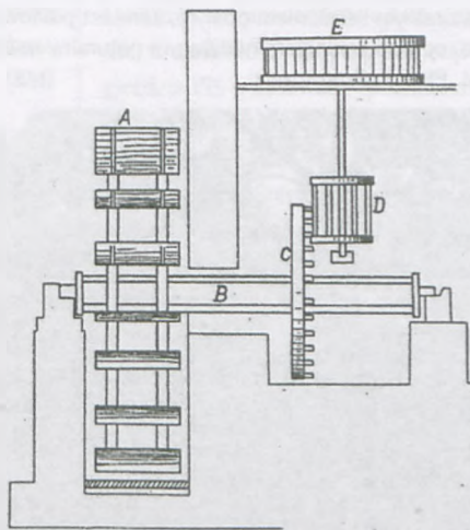
Schemat średniowiecznego młyna wodnego:
