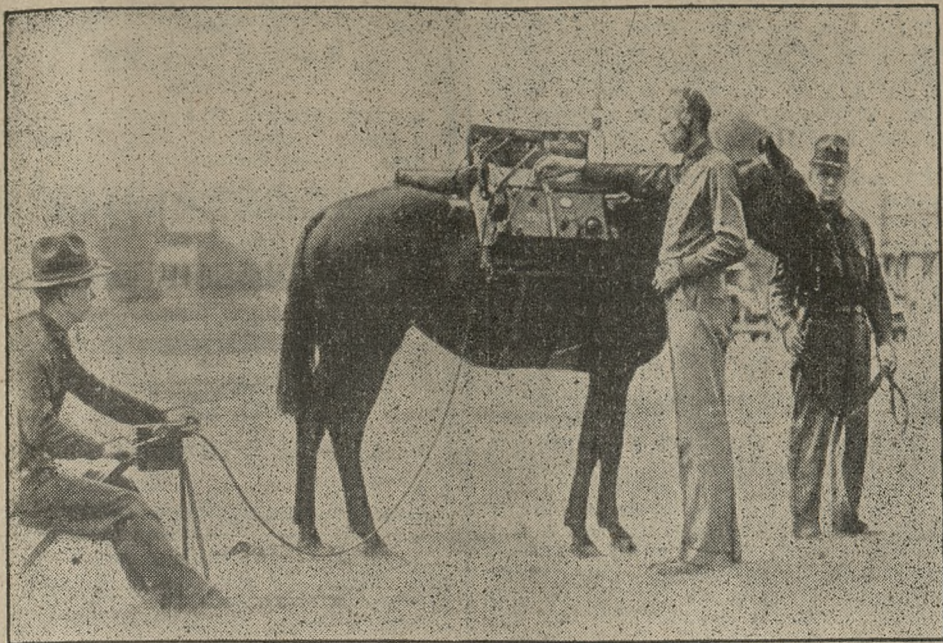
Świeżo została skonstruowana pierwsza radjostacja konna. Gdzie? Oczywiście w Ameryce, w forcie Monmouth, położonym w stanie New Jersey. Energję potrzebną do nadawania wiadomości wytwarza się przy pomocy małego generatora ręcznego, jak to widzimy na zdjęciu z lewej strony.
