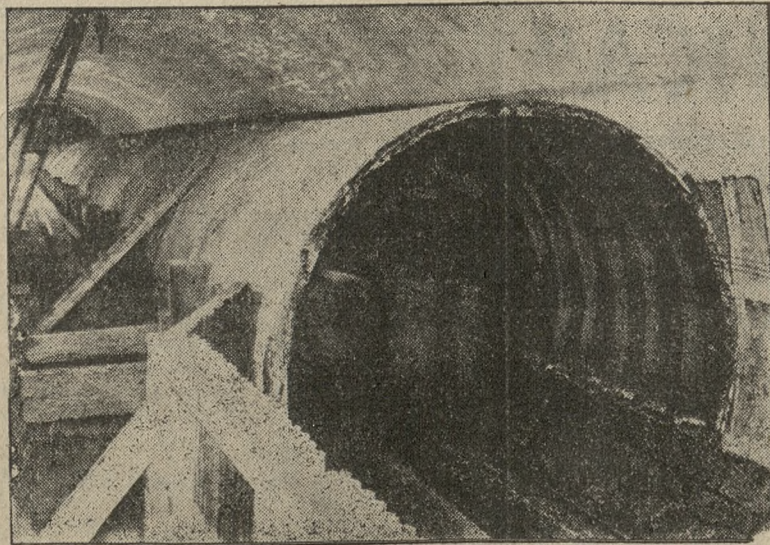
Tunel dokoła tunelu. W Londynie dawny tunel kolei podmiejskiej już nie wystarcza. Trzeba go było rozszerzyć. Ale jak? Pomysłowy inżynier orzeprzawdził więc budowę nowego tunelu dokoła tunelu dawnego, tak że w czasie robót ruch komunikacyjny podmiejski nie doznał ani chwili przerwy. Usunięcie betonu dawnego tunelu nastąpi po zupełnem wykonczeniu nowego.
