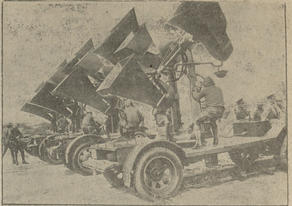
Z manewrów armii amerykańskiej: Bateria najnowocześniejszych aparatów, sygnalizujących najazd samolotów w nieprzyjacielskich na bardzo znaczną odległość. Wobec nich będzie to rzeczą niełatwą dla lotników nieprzyjacielskich podkraść się niespostrzeżenie.
