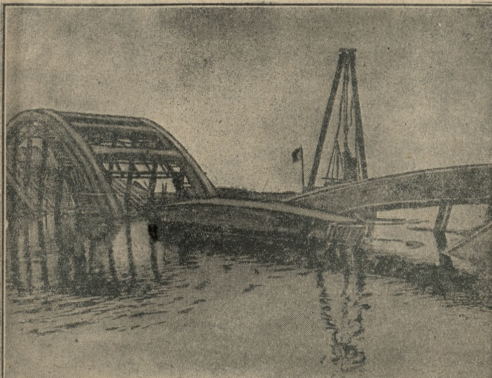
Nowy most betonowy, wzniesiony w Garzu (rej. Szczecińska) na Odrze, miał być oddany do użytku publicznego 26 września b. r. Tymczasem, jak wiadomo, 19 września most uległ katastrofie; cała środkowa część mostu runęła, przyczem 4 robotników poniosło śmierć na miejscu. Rycina nasza przedstawia most po katastrofie.
