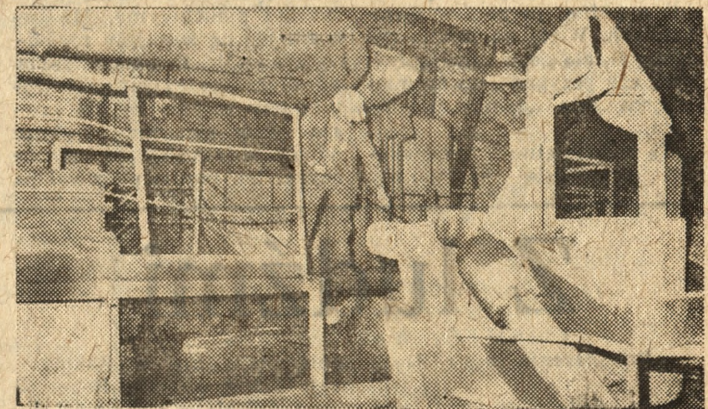
Automatyczna linia do zalewania form w śremskiej odlewni HCP.
