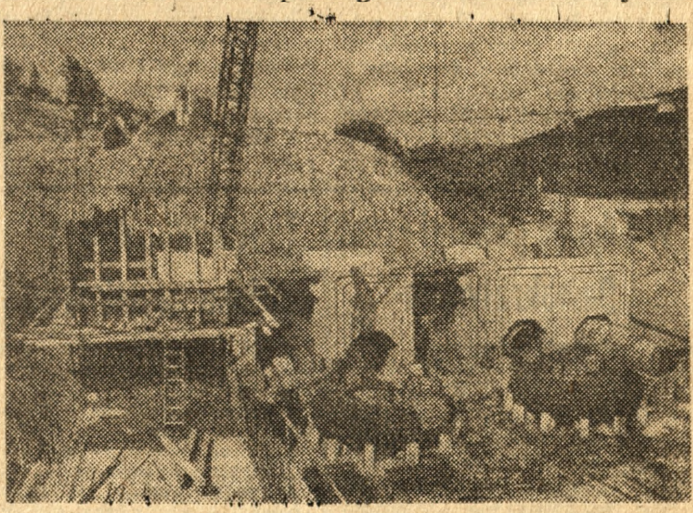
U stóp zamku w Niedzicy koło Czorsztyna trwa budowa zapory na Dunajcu. Obecnie montuje się — przy pomocy specjalistów z Czechosłowacji — elementy turbin rurowiczkowych i energetycznych. Praca ta wymaga dużej precyzji. Na zdjęciu: fragment placu budowy.
