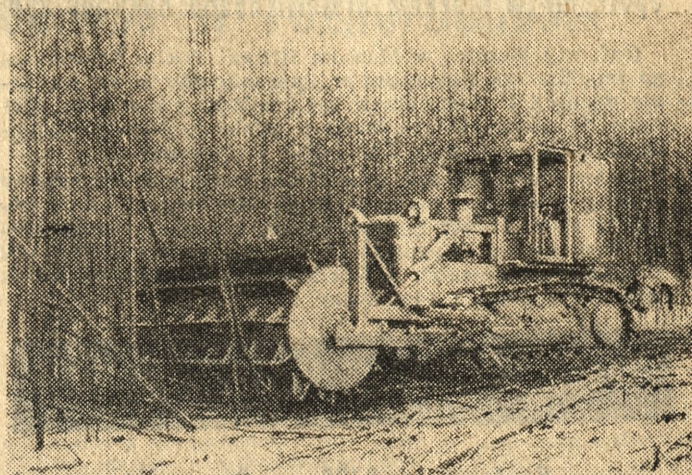
Zielonogórcy inżynierowie skonstruowali zgniatarkę do drzew, którą wykorzystuje się do usuwania z lasów drzew zniszczonych przez pożary i przez brudnicę-mniszkę.
