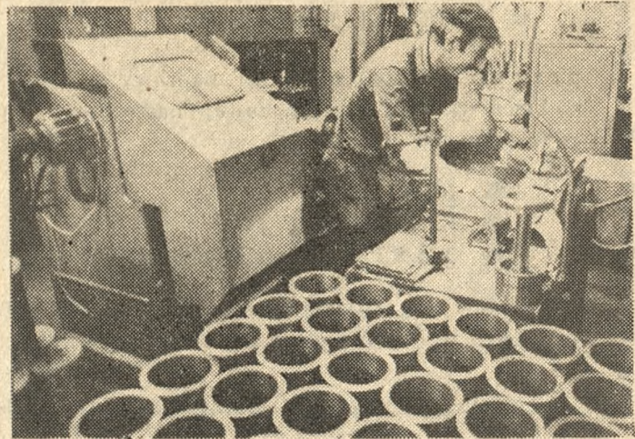
Wszystkie w kraju wytwórnie silników i stacje „Polmozybytu” otrzymują z Krotosyna (Kaliskie) odpowiednie tuleje cylindrowe. Wyabia się je w tamtejszej Wytwórni Sprzętu Mechanicznego. Na zdjęciu: Henryk Wojciechowski przy pomiarach toczonych elementów.
