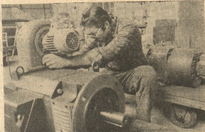
Warsztat produkcji doświadczalnej w Wielkopolskiej Fabryce Maszyn Elektrycznych „Ema — Wielam” przygotowujący przyszłościową produkcję zakładu, rozpoczął montaż pierwszych silników elektrycznych prądu stałego na licencji firmy „Telefunken”. Na zdjęciu: Marek Dolata montuje układ chłodzący silnika. Fot. R. Krolak
