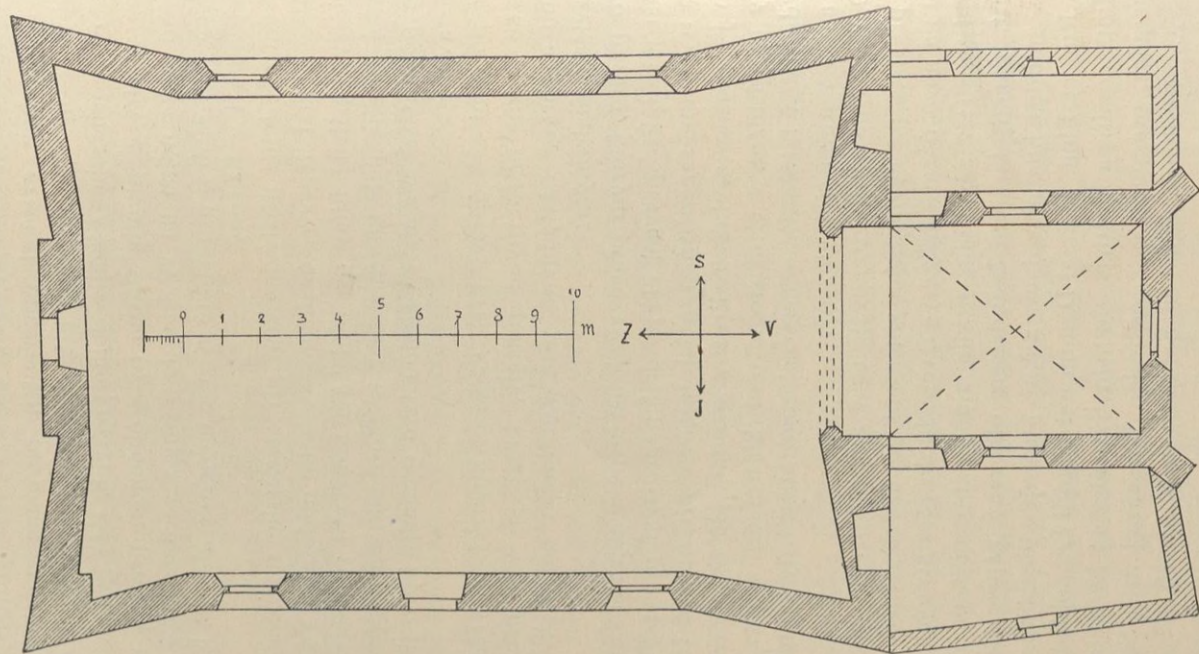
Obr. 33. Půdorys kostela sv. Markety. Rýsoval Jos. Braniš.
