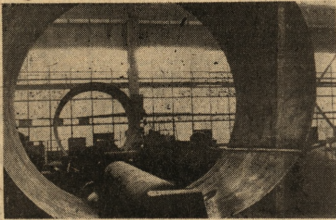
Zakłady Urządzeń Chemicznych „Metalchem” w Kościanie (Leszczyńskie) produkują różne zbiorniki i cysterny. Dzięki specjalnym przyrządom gnie się blachę, tworząc ściany zbiorników. Przygotowanie kolejnych — przedstawia zdjęcie.
