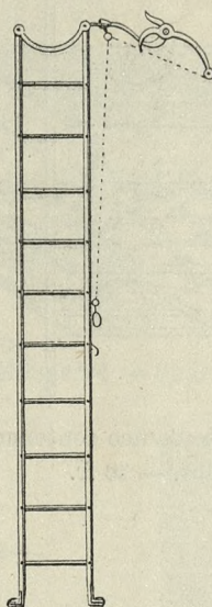
N° 44. — Echelle à sécateur.
