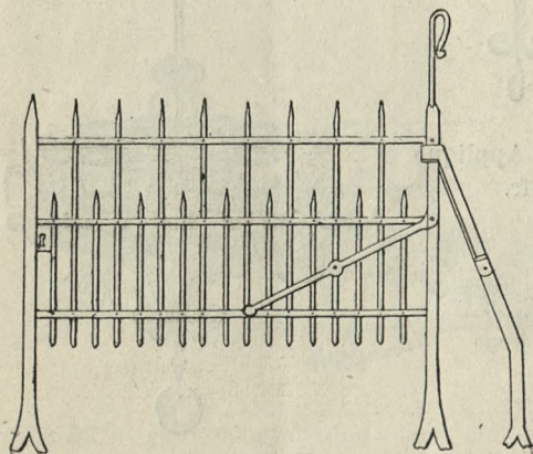
N° 23. — Barrière pont-levis.
