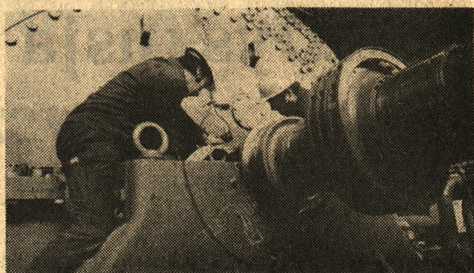
W elektrowni „Połaniec” (woj. tarnobrzezkie) pracują trzy bloki zasilające sieć krajową. Trwa budowa kolejnych bloków. Na zdjęciu: pracownicy Energomontażu Południe dopasowują łożyska uszczelniające generatora bloku IV. CAF — fot. Stan
