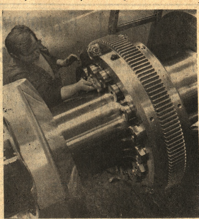
Zakłady Przemysłu Metalowego H. Cegielski w Poznaniu utrzymują rytmiczną produkcję, dostarczając wyroby dla gospodarki krajowej i odbiorców zagranicznych. Na zdjęciu: przygotowanie wału korbowego do montażu w hali Fabryki Silników Okrętowych.
