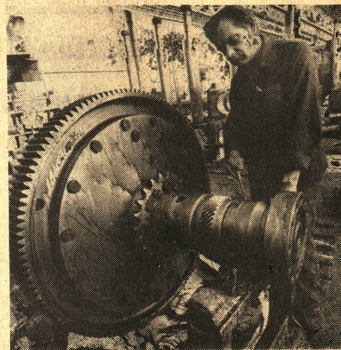
Fabryka Silników Okrętowych Zakładów Przemysłu Metalowego H. Cegielski w Poznaniu mimo sezonu urlopowego pracuje na pełnych obrotach. Miesięcznie wykonuje się tutaj średnio cztery silniki, przeznaczone dla statków, budowanych w naszych stoczniach; część trafia również do odbiorców za granicą. Na zdjęciu: konserwacja elementów silnika.
