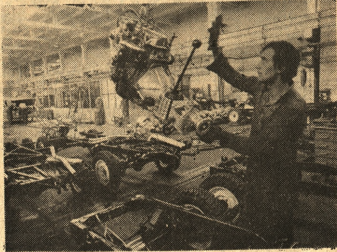
Montaż silnika w poznańskim zakładzie Fabryki Samochodów Rolniczych „Polmo”, która produkuje także na eksport. W minio- nym półroczu wyeksportowano 116 „Tarpanów”. Fot. — R. Królak
