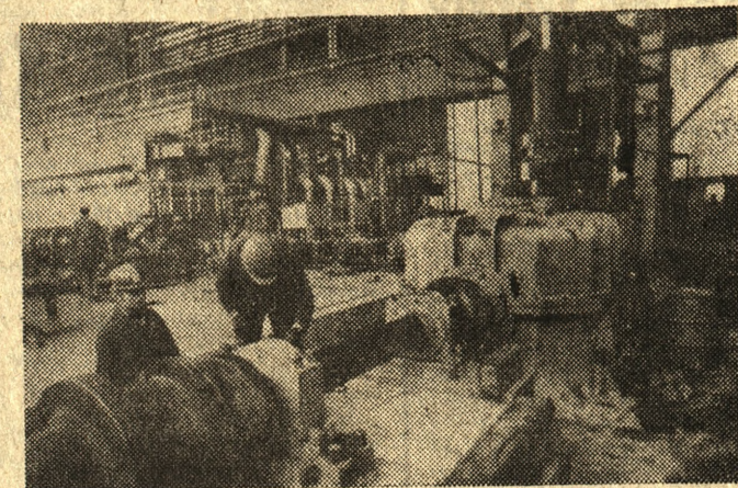
Budowa walcowni drobnej w Hucie im. Nowotki w Ostrowcu Świętokrzyskim jest drugim po Hucie „Katowice” placem budowy w naszym przemyśle metalurgicznym. Ostrowiecka „drobna” będzie największym tego typu obiektem w Europie. Na zdjęciu: montaż urządzeń w hali głównej.
