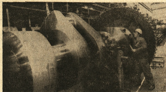
Fabryka Silników Okrętowych poznańskich Zakładów Przemysłu Metalowego H. Cegielski wyprodukowaniem 11 silników wykonana plan kwartalny. Na zdjęciu: montaż korbowodu do silnika przeznaczonego dla francuskiego odbiorcy. CAF — fot. Staszyszyn
