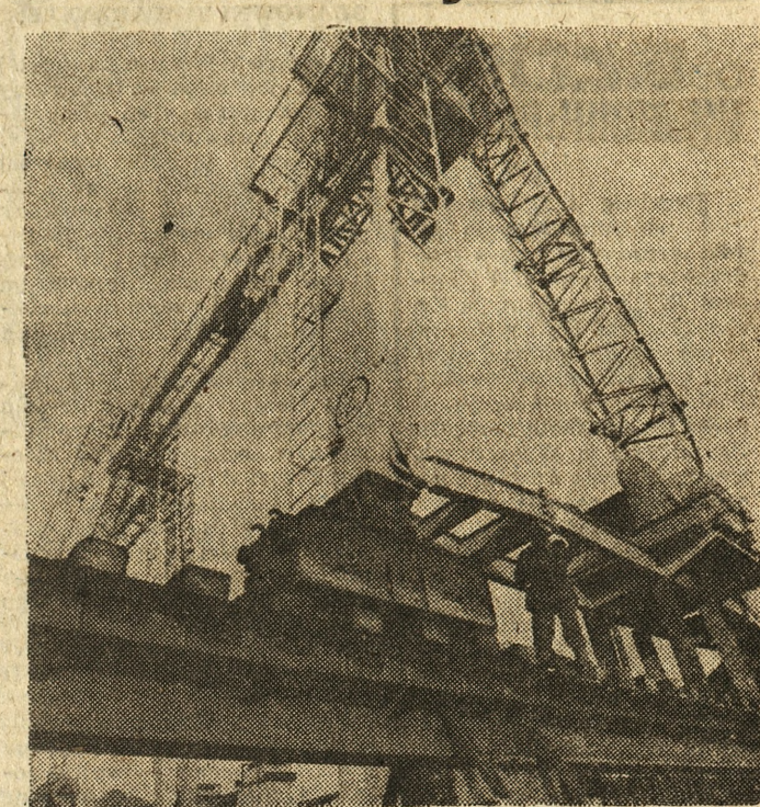
Podczas robót przy kolejnej stołecznej arterii komunikacyjnej — Trasie Toruńskiej — prace koncentrują się obecnie przy wznoszeniu mostu na Wiśle. Zimowa pogoda nie powoduje przerw w budowie.
