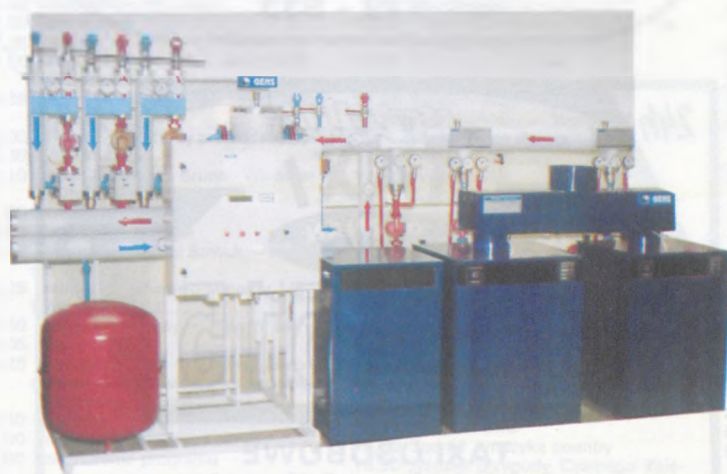
CENTRALE GRZEWcze DWUFUNKCYJNE dla budo- wnictwa wielorodzinnego, budynków użyteczności pu- blicznej i zakładów pracy
