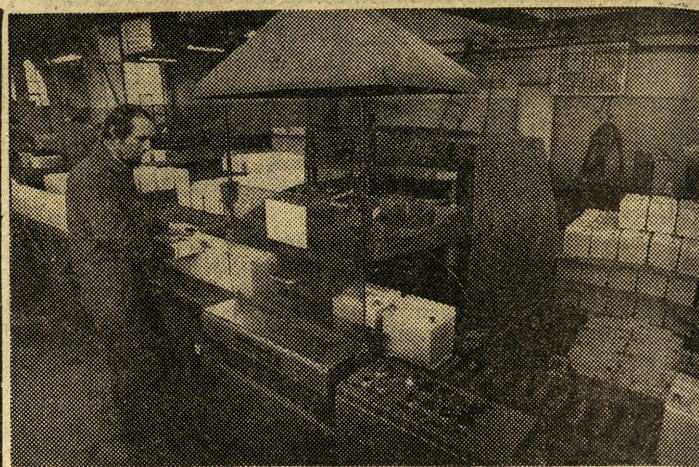
Poznańskie Zakłady Elektrochemiczne „Centra”: linia do zgrzewania akumulatorów 45 Ah.
