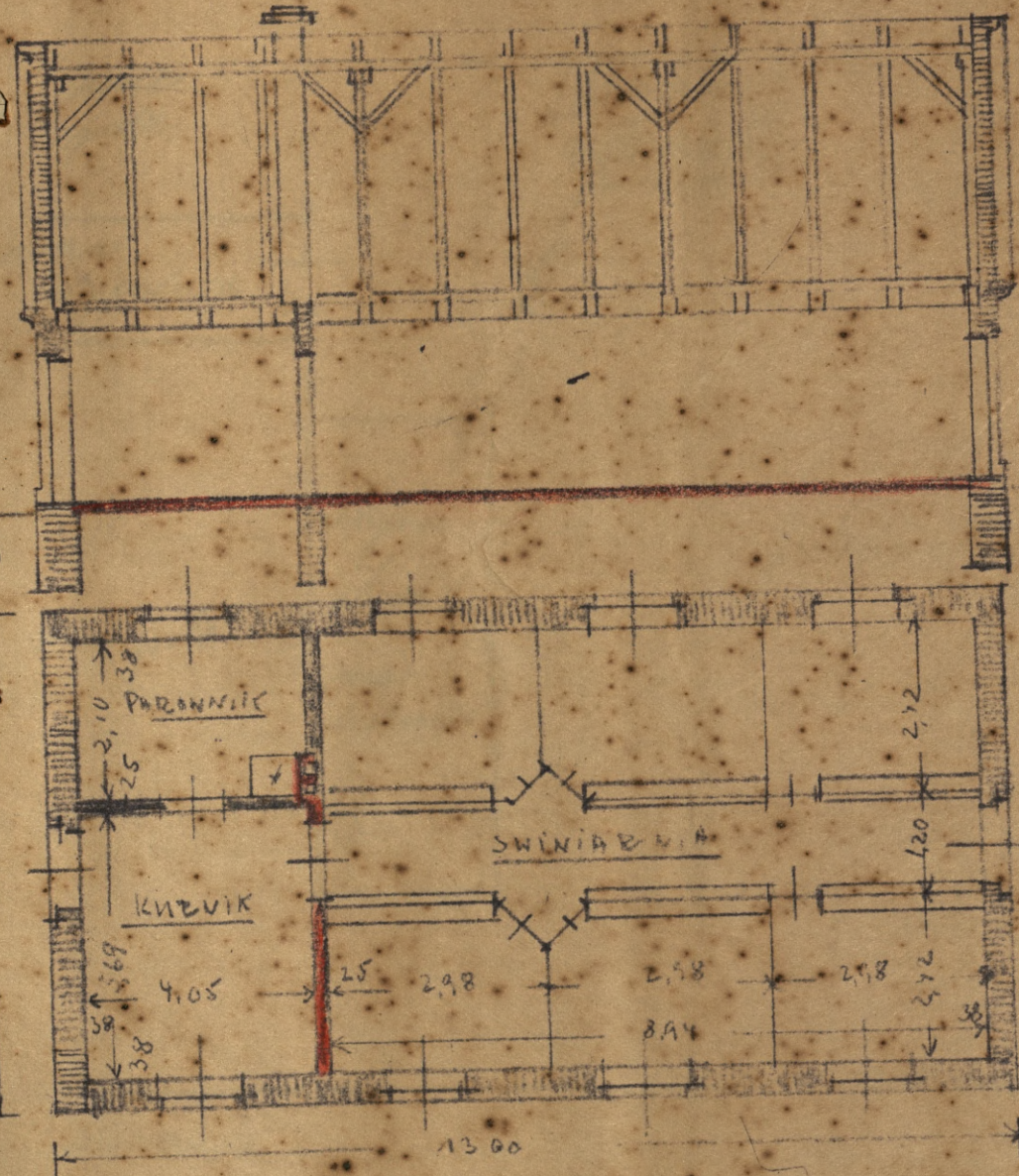
Plan poziomy
