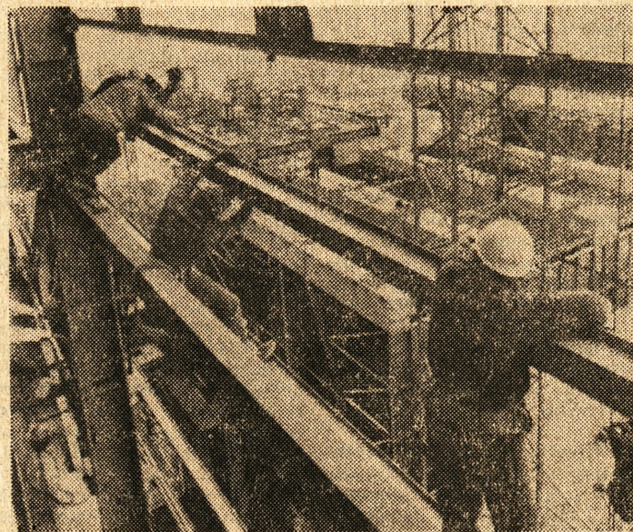
W Potańcu (woj. tarnobrzeskie) powstaje kolejna elektrownia. Będzie ona w przyszłości dostarczać krajowi 1600 MW. Na zdjęciu: montaż ścian osłonowych budynku głównego elektrowni.
