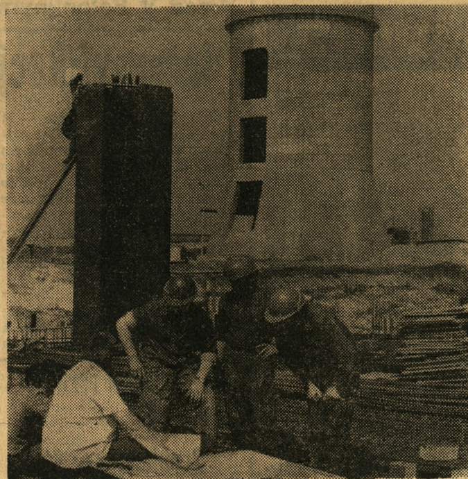
11 firm specjalistycznych pracuje przy budowie elektrowni „Opole”. Obecnie główne prace koncentrują się przy wznoszeniu komina, chłodni oraz budynku głównego. Pierwszy prąd z „Opola” powinien popłynąć w 1981 roku.
