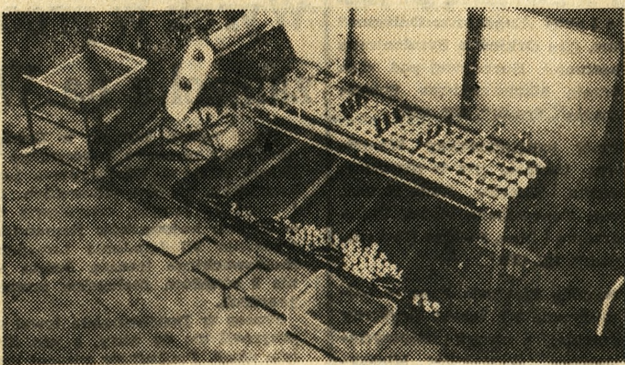
Na zdjęciu: Sortownik diafragmowy do pomidorów o wydajności 5 ton na godzinę.
