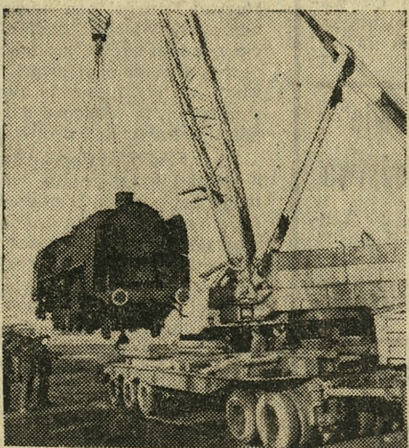
Za chwilę dźwig ustawi parowóz na przyczepie samochodowej. Fot. — R. Królik
