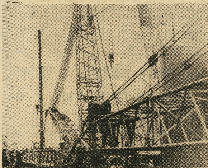
Ten samojezdny dźwig-kołos unosi ciężar do 250 ton, na wysokość 90 metrów. Dzięki niemu akcja usuwania szkód w elektrowni „Adamów” będzie o wiele dni krótsza.
