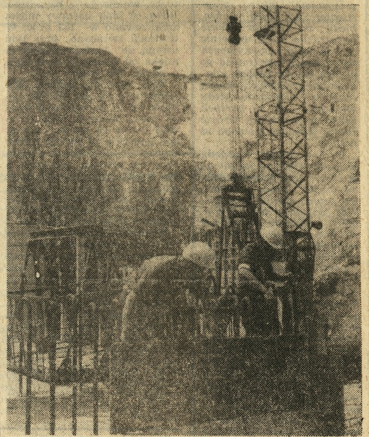
Na Dunajcu koło Czorsztyna powstaje zbiornik wodny o pojemności 250 milionów metrów sześciennych. Zbiornik ten obok zadań przeciwpowodziowych, w razie potrzeby będzie zasilał w wodę elektrownię Potaniec. Na zdjęciu: budowa wlotów do szluciny energetycznych. CAF — fot. Motot
