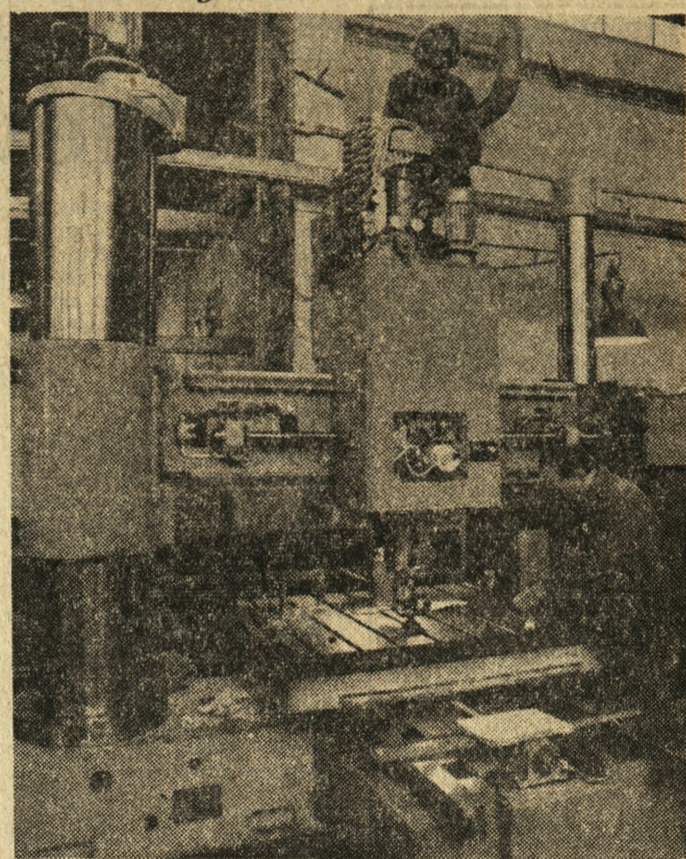
Jednym z potentatów naszego przemysłu maszynowego jest Fabryka Obrabiarek ZPM „H. Cegielski” w Poznaniu. Zakład produkuje kilka odmian automatów tokarskich, a także wiertarki i tokarki sterowane numerycznie. Na zdjęciu — podczas montażu wspomnianej wiertarki. CAF — fot. Rosiak
