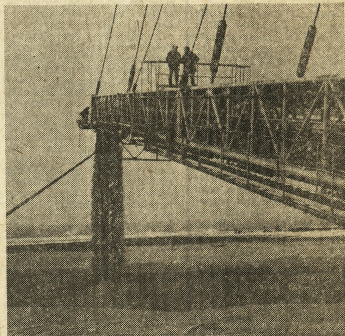
W Kopalni Węgla Brunatnego w Bełchatowie wydobyto już ponad 16 mln metrów sześciennych nadkładu, przykrywającego złoża węgla. Na zdjęciu: gigantyczna zwalowarka.
