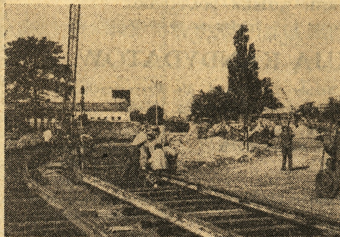
Na przebudowywanym skrzyżowaniu ulic Towarowej i Gwardii Ludowej, brygady poznańskiego „EnergoPolu” rozpoczęły wczoraj wzbijanie katarfem kilkumetrowych pał konstrukcji tunelu, a ekipy WPK układają nowe torowisko.
