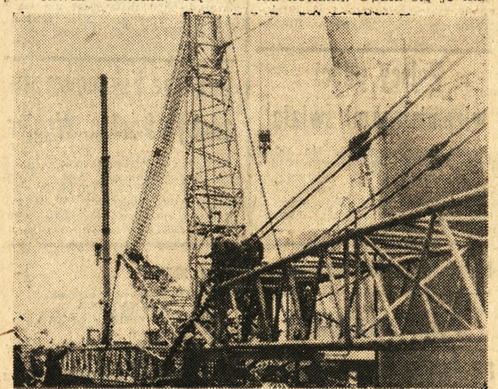
Ten samojezdny dźwig-kolos unosi ciężar do 250 ton, na wysokość 90 metrów. Dzięki niemu akcja usuwania szkód w elektrowni „Adamów” będzie o wiele dni krótsza.
