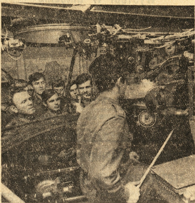
Pod okiem doświadczonych wykładowców podchorążowie Wyższej Szkoły Oficerskiej Wojsk Pancernych im. Stefana Czarnieckiego w Poznaniu zdobywają umiejętności w posługiwaniu się poszczególnymi mechanizmami czołgu.
