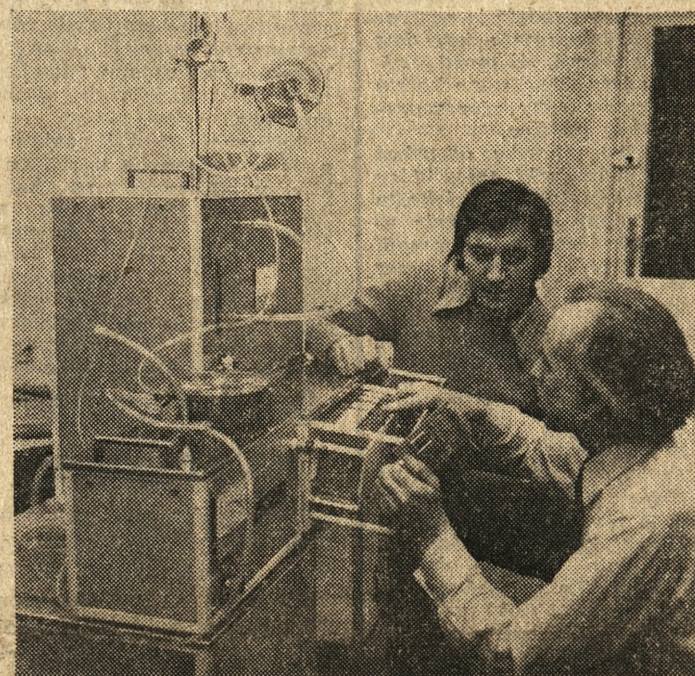
W Zakładach Elektronicznej Aparatury Medycznej w Zabrze rozpoczęto seryjną produkcję aparatu zwanego „szluzką nerką”. Pierwszą serię 25 aparatów otrzyma krajowa służba zdrowia. Na zdjęciu — podczas prób uruchamiania. CAF — fot. Jakubowski
