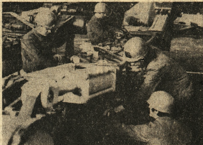
Piotrowicka Fabryka Maszyn „Famur” jest producentem ścianowych kombajnów węglowych. Plan na rok bieżący przewiduje 200 tego typu maszyn. Na zdjęciu: podczas montażu kombajnu. CAP — fot. Seko
