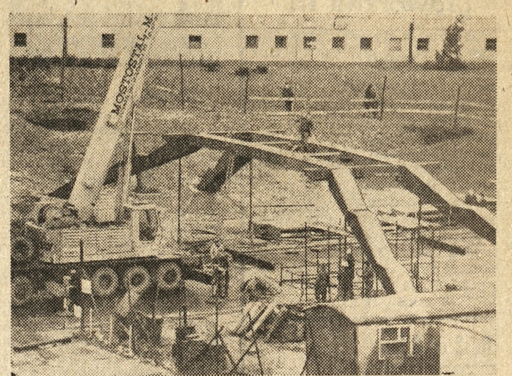
Oto rezultat trwającego od Gwiazdki do Sylwestra montażu kładki dla pieszych przy ul. Słowiańskiej. Wczoraj ulica nadal była zamknięta dla ruchu przelotowego, chociaż oficjalny komunikat zapowiadał jej zamknięcie w dniach od 27 do 31 grudnia.
