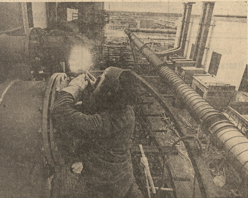
Pod Głogowem dobiega końca budowa drugiej huty miedzi. Trwają ostatnie prace montażowe w tlenowni oraz w części zwanej ogniową. Roboty wykonują specjaliści wielu krajowych przedsiębiorstw. Na zdjęciu: spawacz Kazimierz Maciejewski z poznańskiego „Mostostalu” montuje instalację rurową tlenowni.
