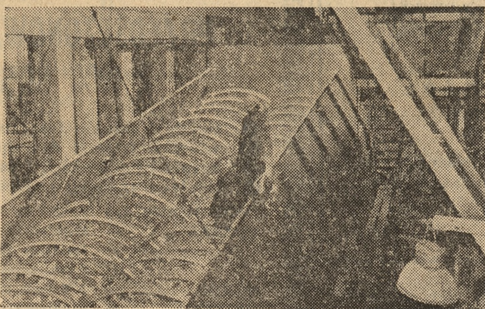
Na zdjęciu: spawacz Kazimierz Adamski w czasie pracy przy no-wym dyfuzorze. Fot. — H. Kamza
