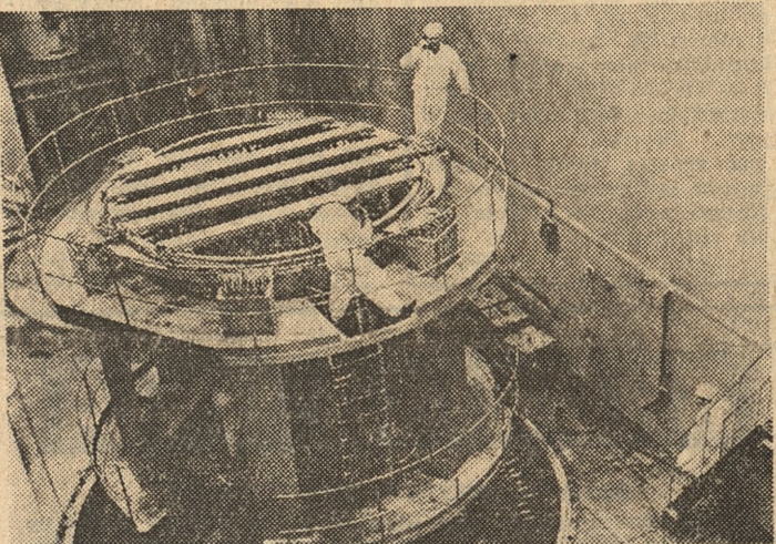
Nowovoroneńska elektrownia atomowa nad Donem zaliczana jest do największych w świecie. Na zdjęciu: hala reaktora drugiego bloku energetycznego.
