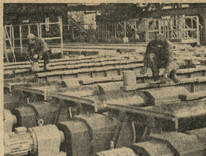
W Hucie im. Nowotki w Osnowcu Świętokrzyskim (woj. kielecki) powstaje nowoczesny wydział ciągłego odlewania stali. Obecnie trwają ostatnie prace montażowe, a także regulacja poszczególnych urządzeń. Na zdjęciu: ostatnie przeglądy transportów w strefie spychacza wlewków w siłowniach. Fot. — CAF
