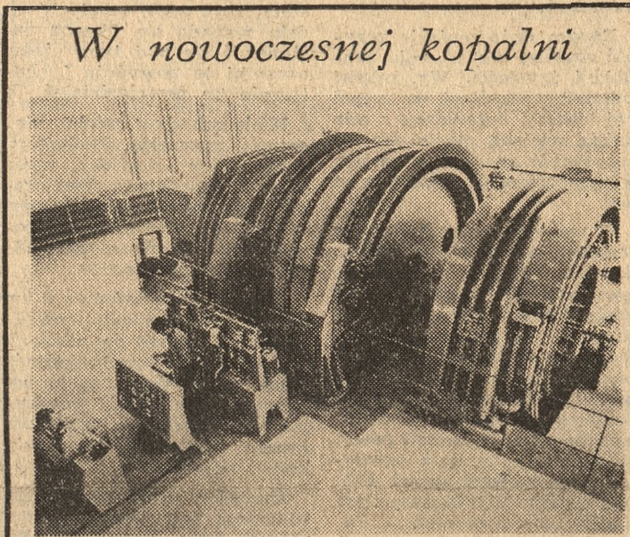
Kopalnia Jankowice należąca do Rybnickiego Okręgu Węglowego ma nowe urządzenie wyciągowe o mocy 2x2900 kW. Ogromna nowoczesna maszyna umożliwi osiągnięcie szybkiego wzrostu wydobywania docelowo do 30 000 ton. Na zdjęciu: kontrola urządzeń maszyny wyciągowej.
