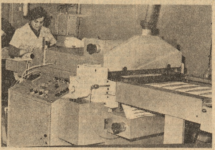
Na tej maszynie-automacie, wyglądającej jak pulpit sterowniczy, zgrzewa się wstęgi z ciasta. Dzięki temu w czasie pracy nie ma odchylenia między kurczliwością ikaniny koszulowej i uszywniającego wkładu. Taka maszyna ze Szwajcarii w ciągu jednej zmiany wykonuje około 12 000 wstęg. Fot. — H. Kamza
