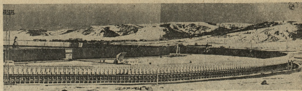
W Astrofizycznym Obserwatorium Akademii Nauk ZSRR, w górach Północnego Kaukazu, znajduje się jeden z największych na świecie radioteleskopów — „Ratan-600”. Średnica jego wynosi 699 metrów. Fot. — CAF
