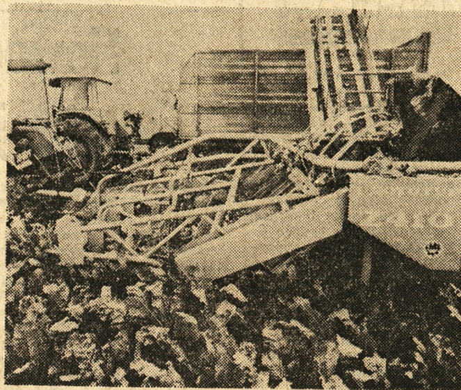
Pracownicy Przemysłowego Instytutu Maszyn Rolniczych w Poznaniu dokonują prób nowego sprzętu. Na polach Stacji Hodowli Roślin w Nagrodzicach koło Poznania pracują nowe maszyny do zbioru buraków cukrowych, konstrukcji słupskiego „Famarolu” i poznańskiego PIMR.
