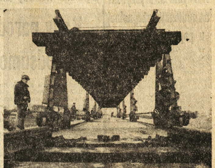
Intensywne roboty trwają przy układaniu toru między Grodziskiem a Włoszczową — na budowie Centralnej Magistrali Kolejowej. Oddanie do wspólnej eksploatacji pierwszej nitki CMK przewiduje się w tym miesiącu. Na zdjęciu: pracownicy poznańskiego PRK 10 układają nowe prześięto toru od strony Grodziska. CAF — fot. — Dąbrowiecki
