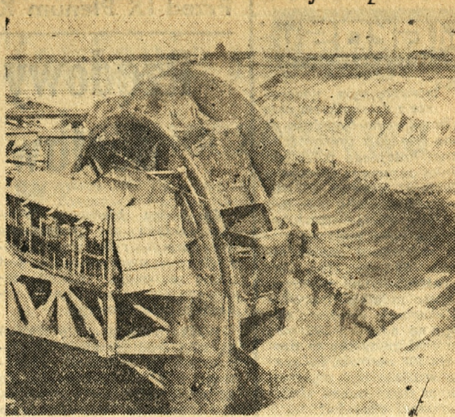
Gigantyczna koparka pracująca w Kopalni Węgla Brunatnego w Bełchatowie zbiera w ciągu doby 100 000 metrów sześciennych nadkładu. Tym samym zbliża się do zdolności docelowej — 110 000 metrów sześciennych.
