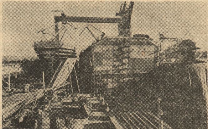
W drugim suchym doku Stoczni im. Komuny Paryskiej w Gdyni trwa budowa pierwszego stalika. Jest to gazowiec typu LPG, prze- znaczony dla armatora zagranicznego. Na zdjęciu: prace przy montażu gazowca. Fot. — CAF
