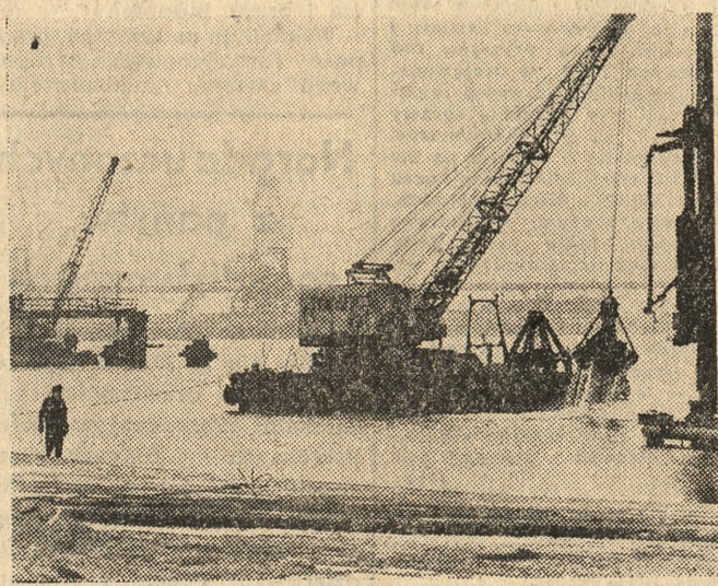
Przy budowie bazy rudy w Porcie Północnym paluje się obecnie teren pod estakady przenośników taśmociągów na pirsie; wykonuje się także ściankę żelbetonową stanowiącą stały brzeg morski. Na zdjęciu: prace katarów przy pirsie rudowym. Fot. — CAF
