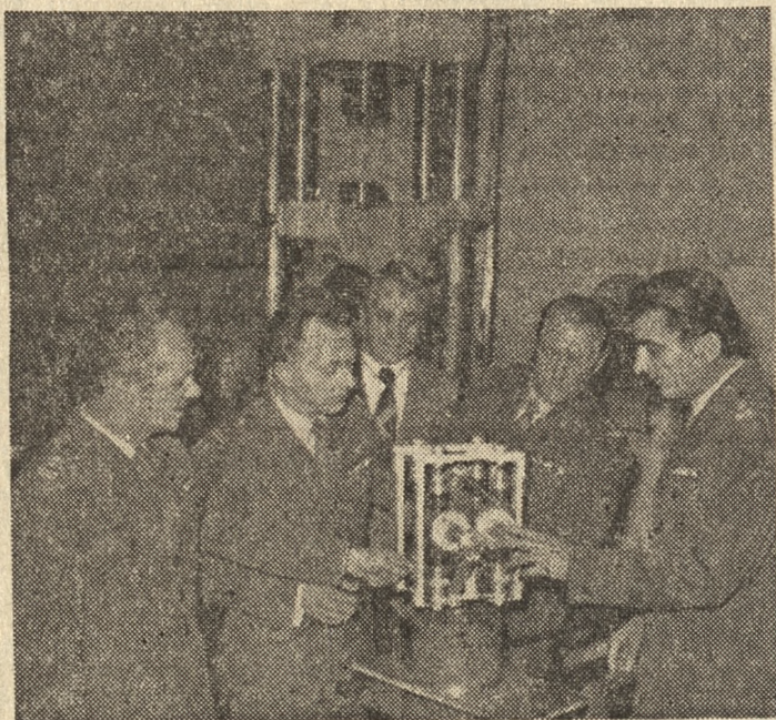
Przy modelu „wibromotu” w Wojskowej Akademii Technicznej. Po raz pierwszy na świecie zastosowano tu jednocześnie działania pionowe i obrotowe - zmienne na zagłębiony element.
